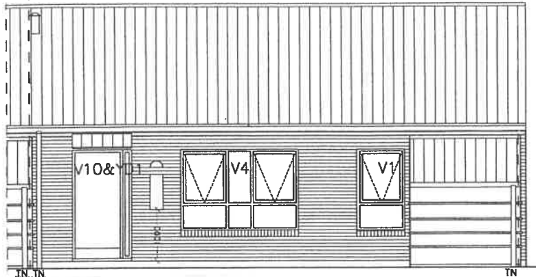
Indgangsfacade, 1:100
