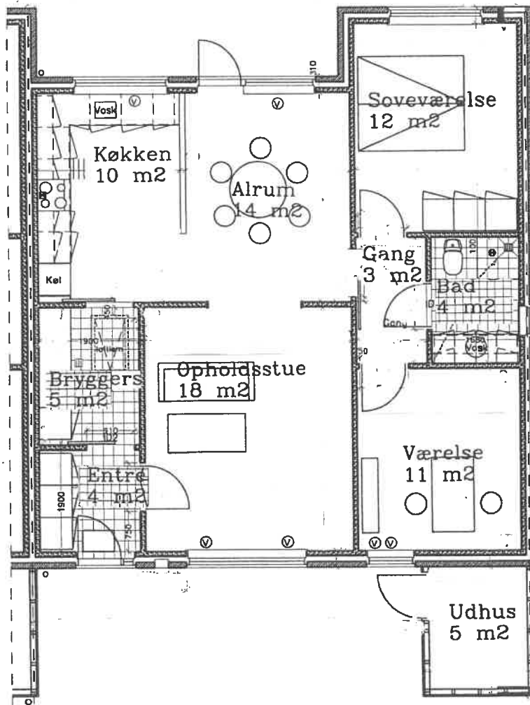
Plan, 1:100
